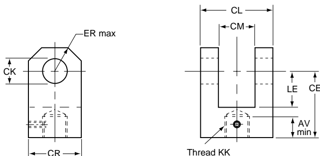
Rod Clevis
